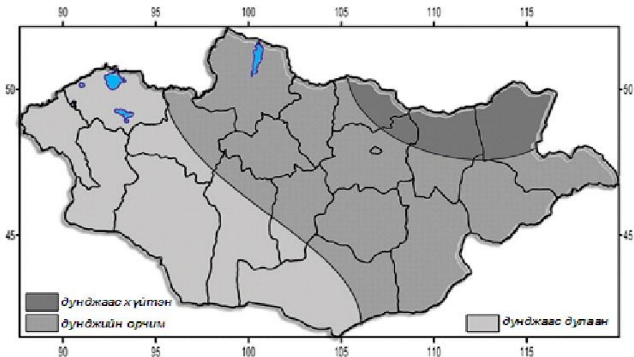
3 дугаар зураг. 11 дүгээр сарын агаарын температурын урьдчилсан мэдээ
