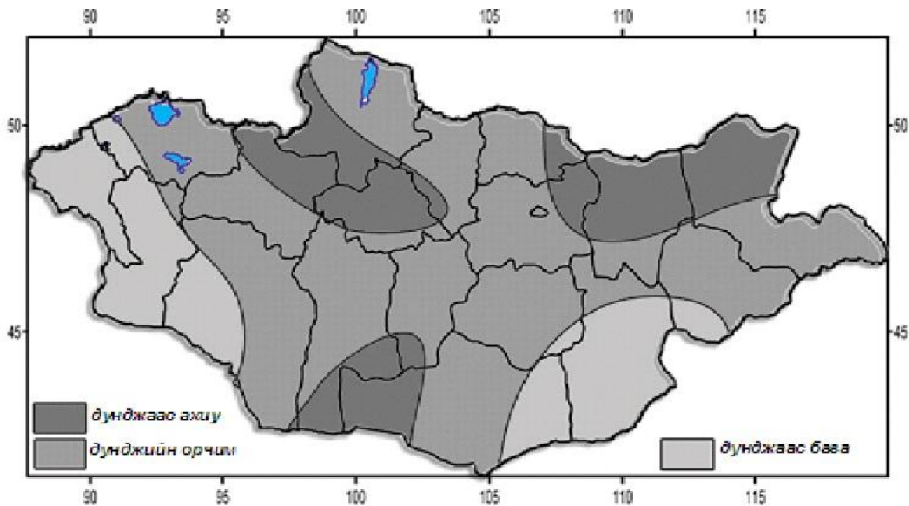
4 дүгээр зураг. 11 дүгээр сард орох хур тунадасны урьдчилсан мэдээ
