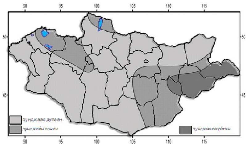
3 дугаар зураг. 1 дүгээр сарын агаарын температурын урьдчилсан мэдээ
