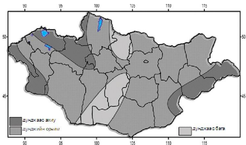
4 дугаар зураг. 1 дүгээр сард орох хур тунадасны урьдчилсан мэдээ
