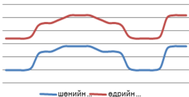
Зураг I.6 2-р сарын агаарын температурын хоногийн явц
